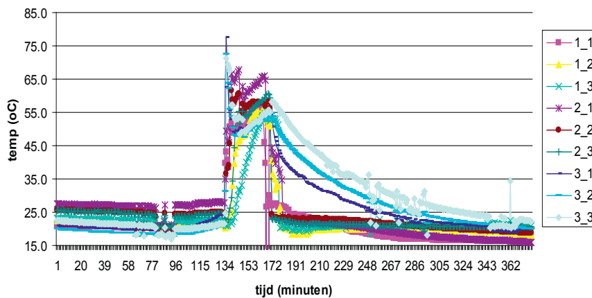
Figuur 11. Temperaturen op drie verschillende locaties en op drie verschillende diepten (1, 7 en 15 cm) in het ondiepe zandbed. De getallen in de legenda geven aan respectievelijk, de locatie in het bed en de dieptes 1=1 cm, 2=7 cm en 3=15 cm.
