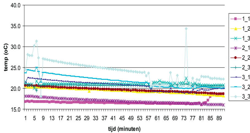
Figuur 10. Temperaturen op drie verschillende locaties en op drie verschillende diepten (1, 35 en 70 cm) in het diepe grondbed. De getallen in de legenda geven aan respectievelijk, de locatie in het bed en de dieptes 1=1 cm, 2=7 cm en 3=15 cm.
