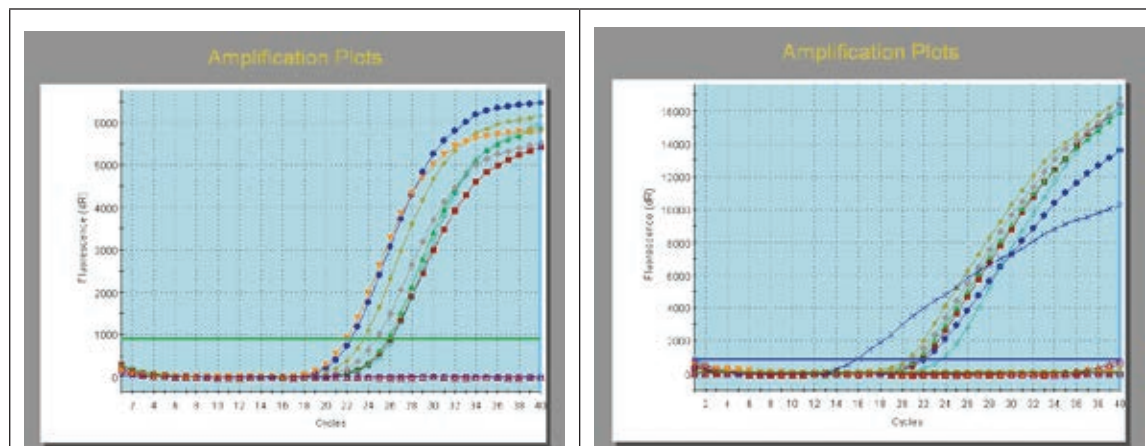
Figuur 11. Amplificatie-curves voor de Trips-PCR. Het aantal cycli waarbij de stijgende S-curve de groene drempelwaarde lijn doorkruist, bepaald de Ct-waarde.
