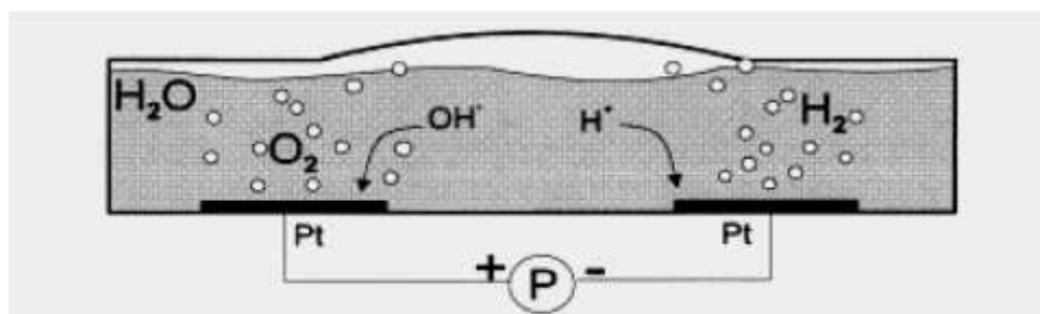
Figuur 1. Schematisch overzicht van een electrochemische cel met water als uitgangspunt (Bron).
