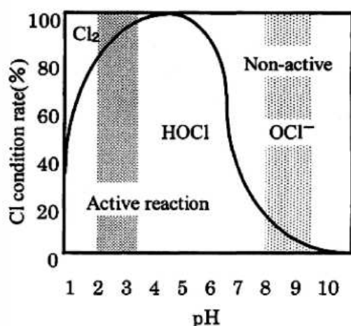
Figuur 4. Het vrij chloor profiel verandert met verschillen in pH. Bij lage pH (2-3) vindt productie van chloorgas plaats en onderchlorig zuur ( \text{HOCl} ), vanaf pH 5 bestaat het merendeel uit onderchlorig zuur en vanaf een neutrale pH vindt vooral omzetting plaats van hypochloriet ( \text{OCl}^- ) (Al haq et al. 2005).
