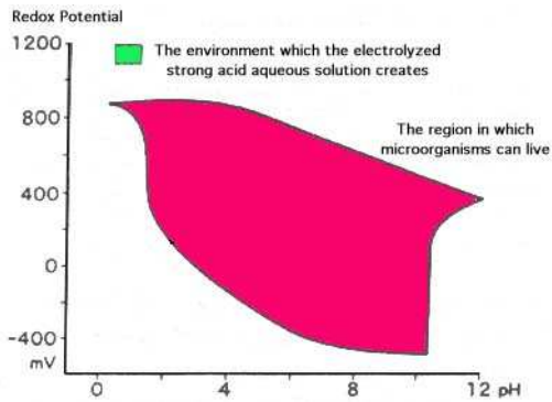
Figuur 5. Figuur laat de invloed van de oxidatie-reductie potentiaal (ORP) en pH van electrochemisch geactiveerd water zien op de bacteriegroei. Bij hoge ORP-waarden boven 800 mV en lage zuurgraad is nagenoeg geen bacterieleven meer mogelijk (Al-Haq et al. 2005).
