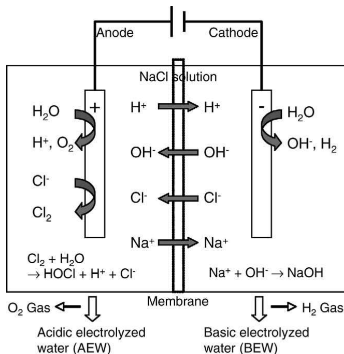
Figuur 2. Schematisch overzicht van een electrochemische cel met een keukenzoutoplossing als uitgangspunt (Hricova et al. 2008, Al-Haq et al. 2005). Tijdens het elektrolyse proces valt een keukenzout ( \text{NaCl} ) oplossing (opgelost in demiwater) uiteen in chloride ( \text{Cl}^- ) en natrium ( \text{Na}^+ ). Hydroxide ( \text{OH}^- ) en waterstof ( \text{H}^+ ) ionen bevinden zich van nature in water. Negatief geladen ionen zoals \text{Cl}^- en \text{OH}^- bewegen zich naar de anode waar de elektronen worden afgegeven en deze zuurstof ( \text{O}_2 ), chloorgas ( \text{Cl}_2 ), hypochloride ion ( \text{OCl}^- ) onderchlorig zuur ( \text{HOCl} ) en zoutzuur ( \text{HCl} ) vormen. Positief geladen ionen zoals \text{H}^+ , gevormd uit de splitsing van water in \text{H}^+ en \text{OH}^- , bewegen zich naar de kathode om elektronen op te nemen en waterstof gas ( \text{H}_2 ) wordt gevormd. \text{OH}^- dat overblijft vormt met het aanwezige \text{Na}^+ opgelost natronloog ( \text{NaOH} ). De oplossing valt uiteen in een zure oplossing van de anode (AEW) met een pH van 2 tot 3, een hoog oxidatie reductie potentiaal (ORP) van >1100 mV, en bevat een hoeveelheid zure, beschikbaar actief chloor van 10 tot 90 ppm, en een basische elektrolyse water oplossing (BEW) van de kathode met een pH van 10 tot 13 en een ORP van -800 tot -900 mV. Het basische water heeft een oppervlaktespanningsverlagende en ontvettende werking.
